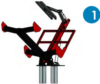
TiltingLift 600 (H-fork)
