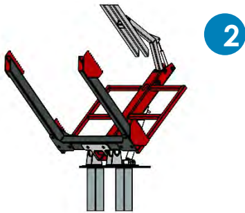
TiltingLift 600 (U-fork)
