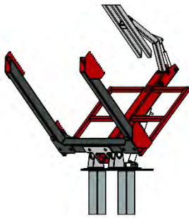
TiltingLift 1800 (U-fork)
